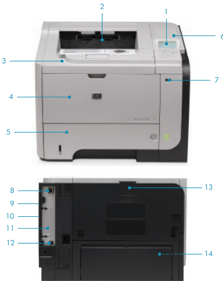
Ilustração da impressora HP LaserJet Enterprise P3015dn
